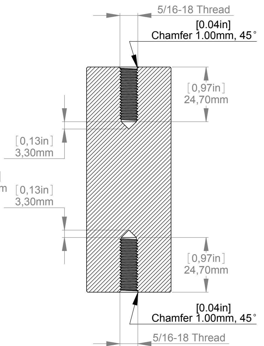
SECTION A-A
