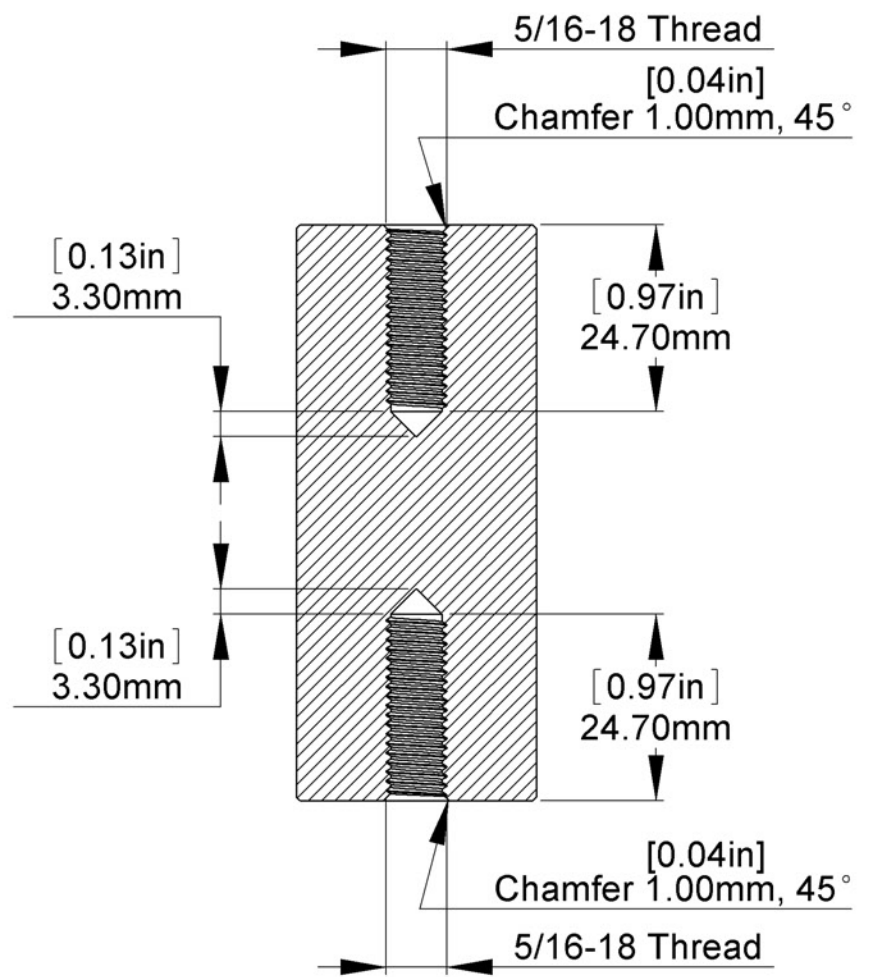
SECTION A-A
