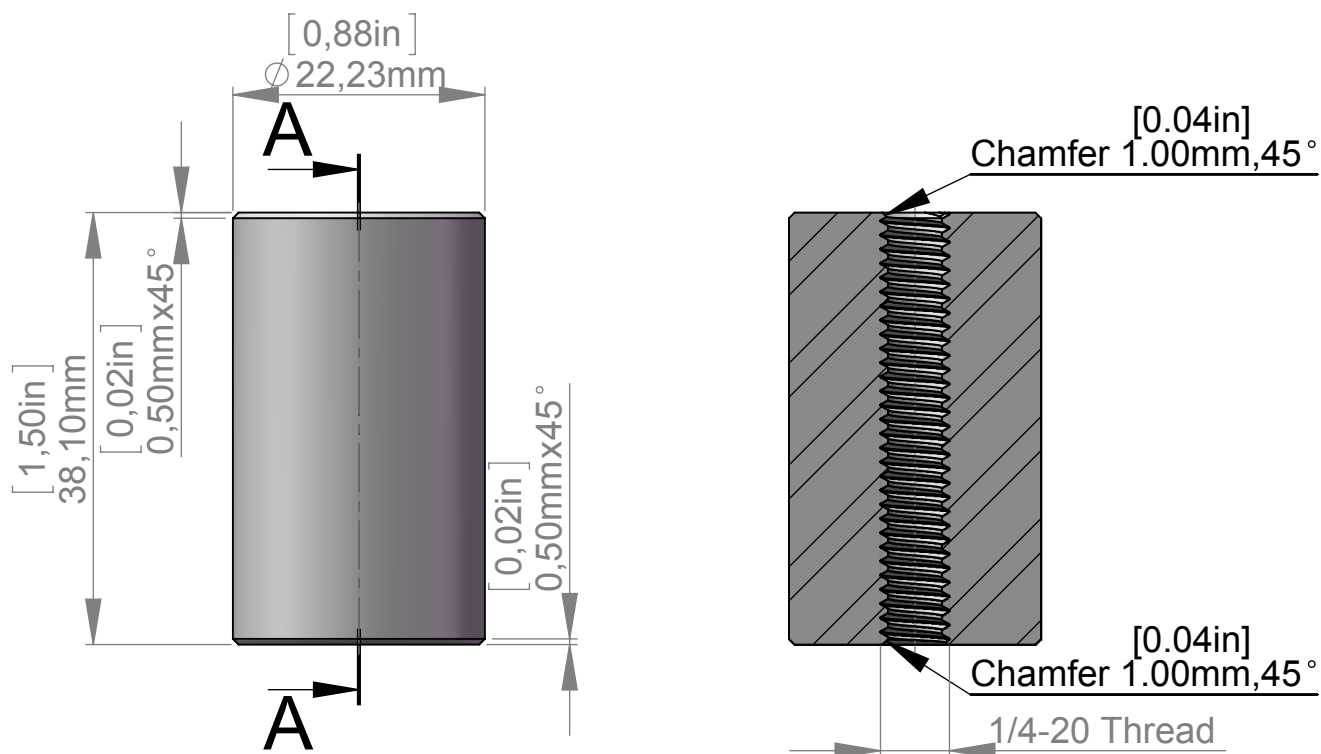
SECTION A-A SCALE 1.5 : 1
