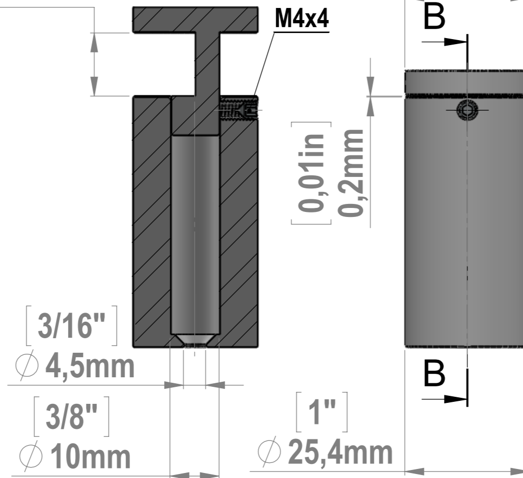
SECTION A-A SCALE 1.3 : 1
