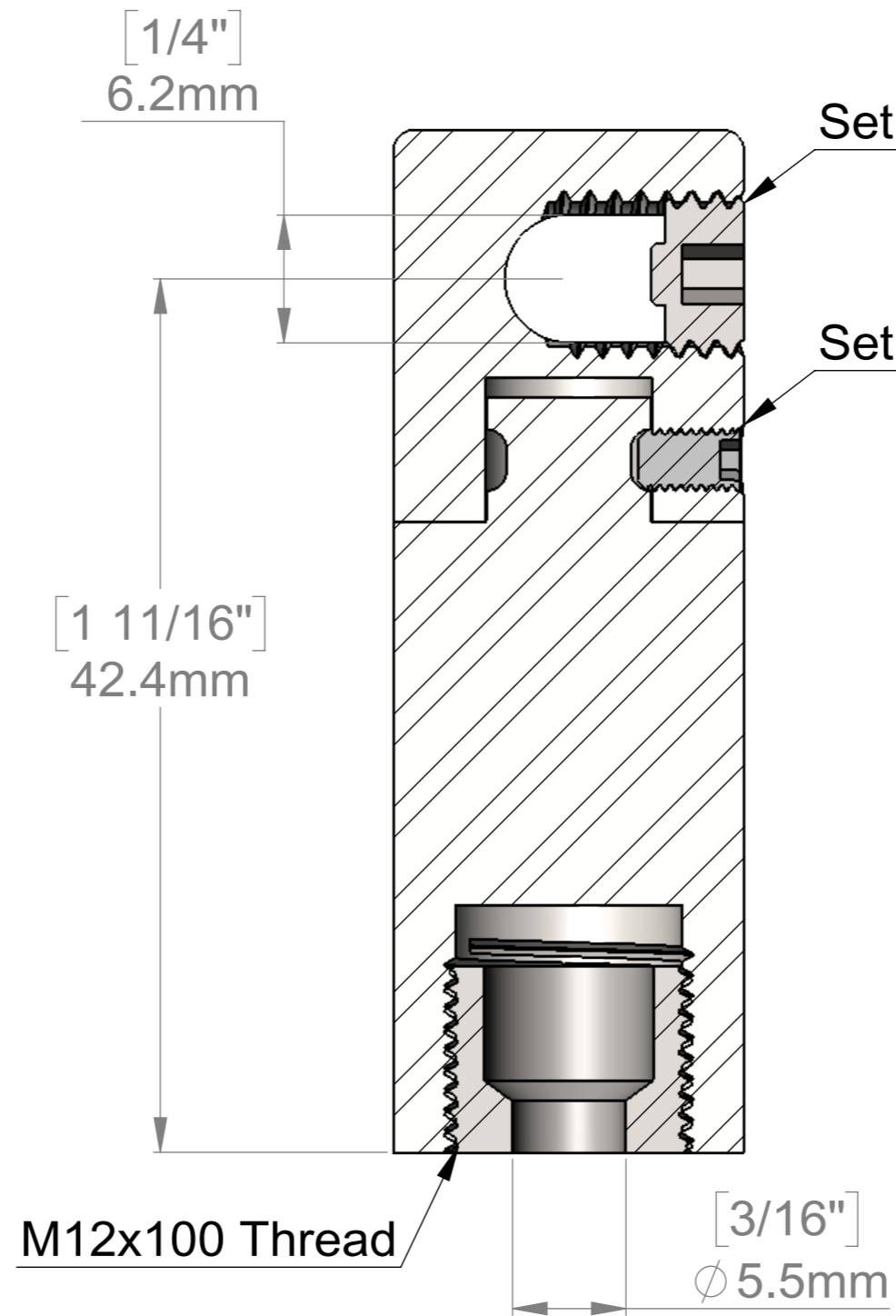
SECTION A-A SCALE 3 : 1
